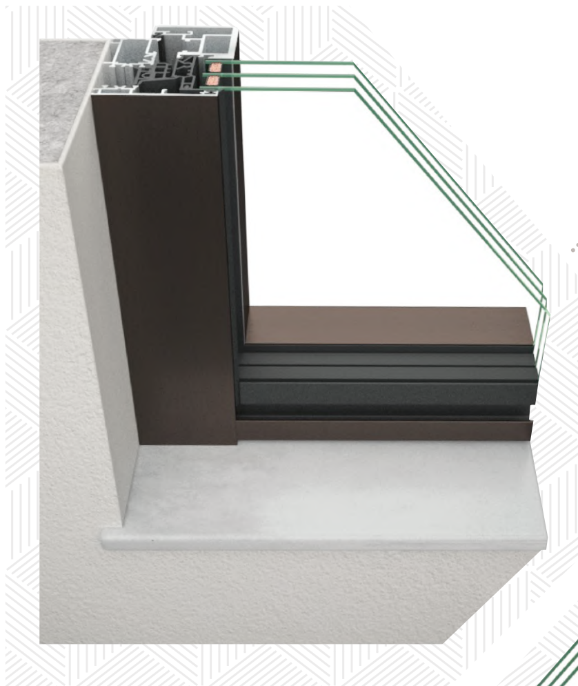
Sistema di posa con telaio a vista
