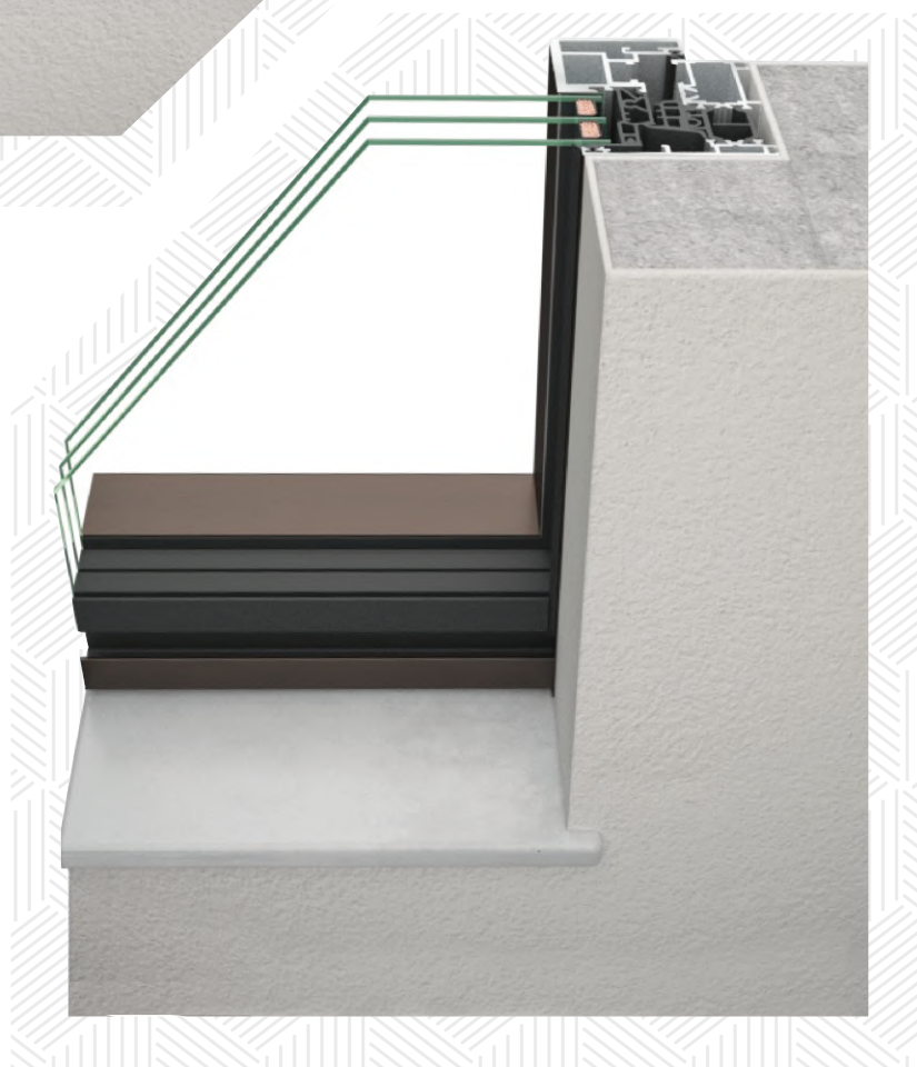
Sistema di posa con telaio a scomparsa
